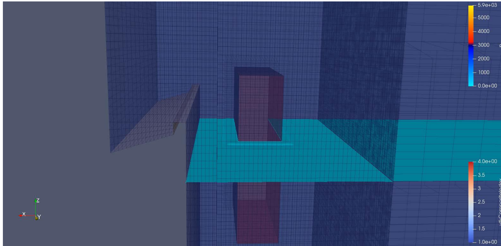
Visualisation de la surface libre pour un essai 3D
